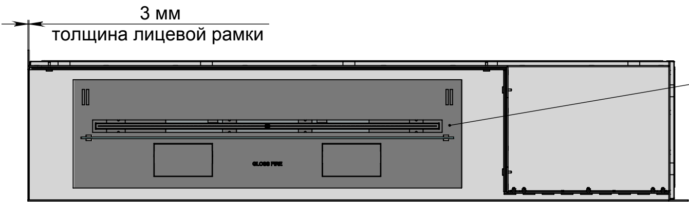
A-A (1 : 10)
