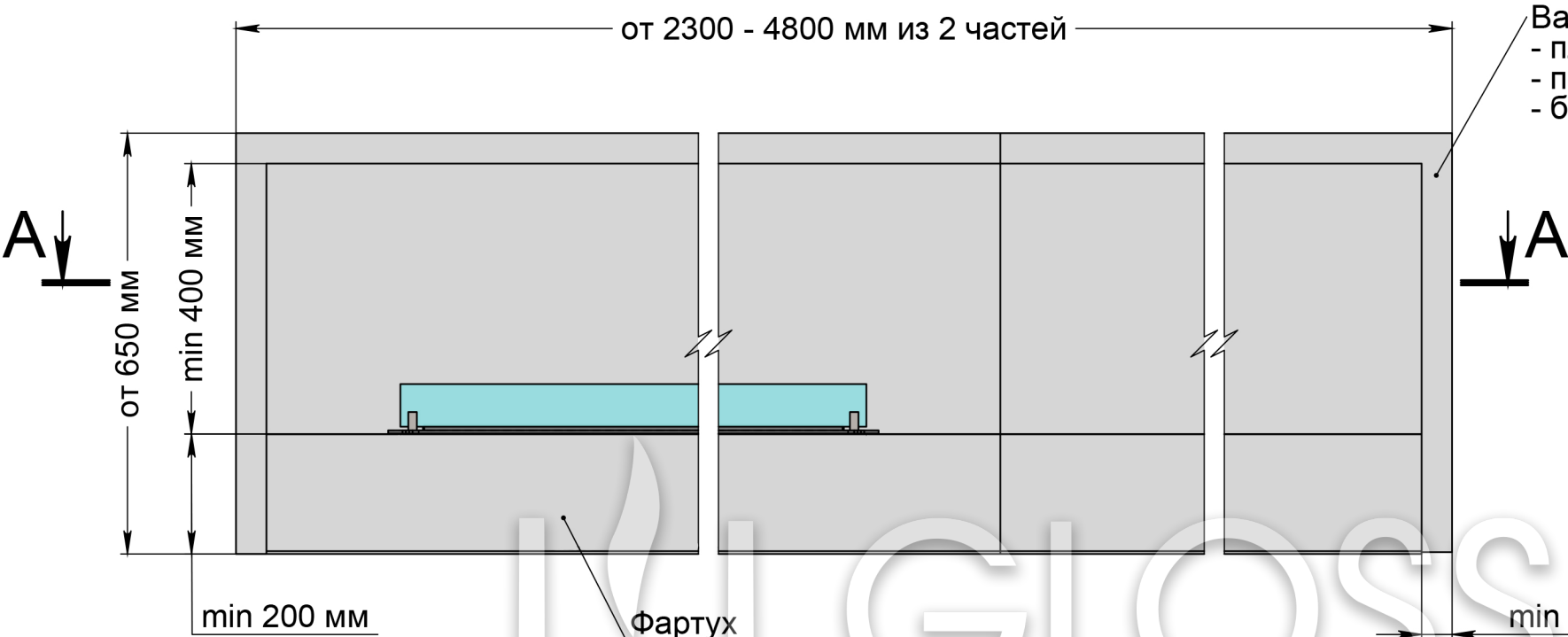
Вид спереди
