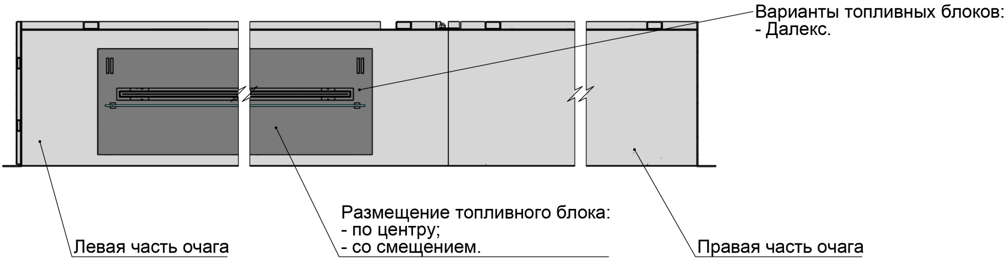
A-A
